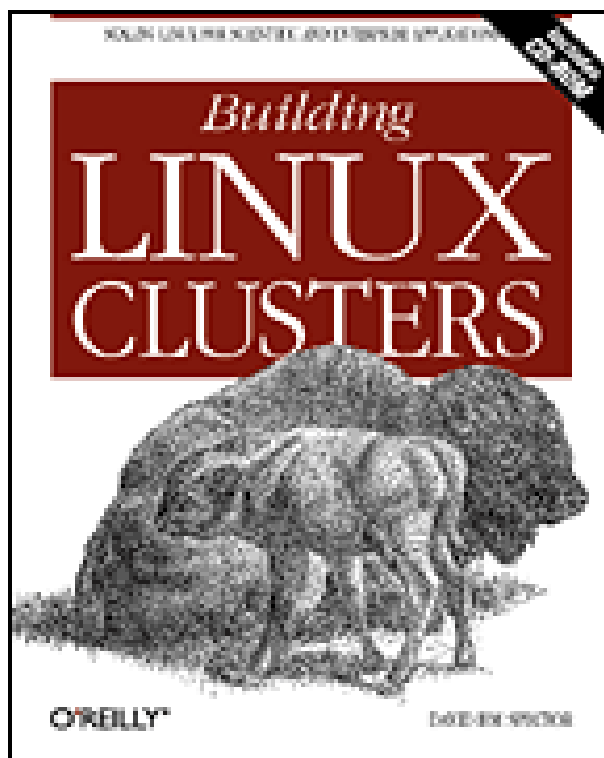
Abbildung 1.1: Linux Clusters
