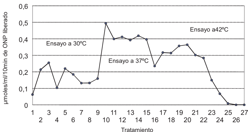
FIGURA 2. μmoles/mL/10min DE ONP LIBERADO vs. LOS NÚMEROS ASIGNADOS A LAS INTERACCIONES, MOSTRANDO EL COMPORTAMIENTO EN BLOQUE DE LOS ENSAYOS POR TEMPERATURA.
